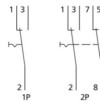
Înterupător-comutator
