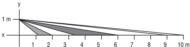
SENKRECHTER DECKUNGSBEREICH
