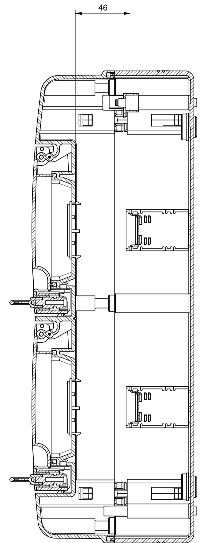
Sezione A-A
