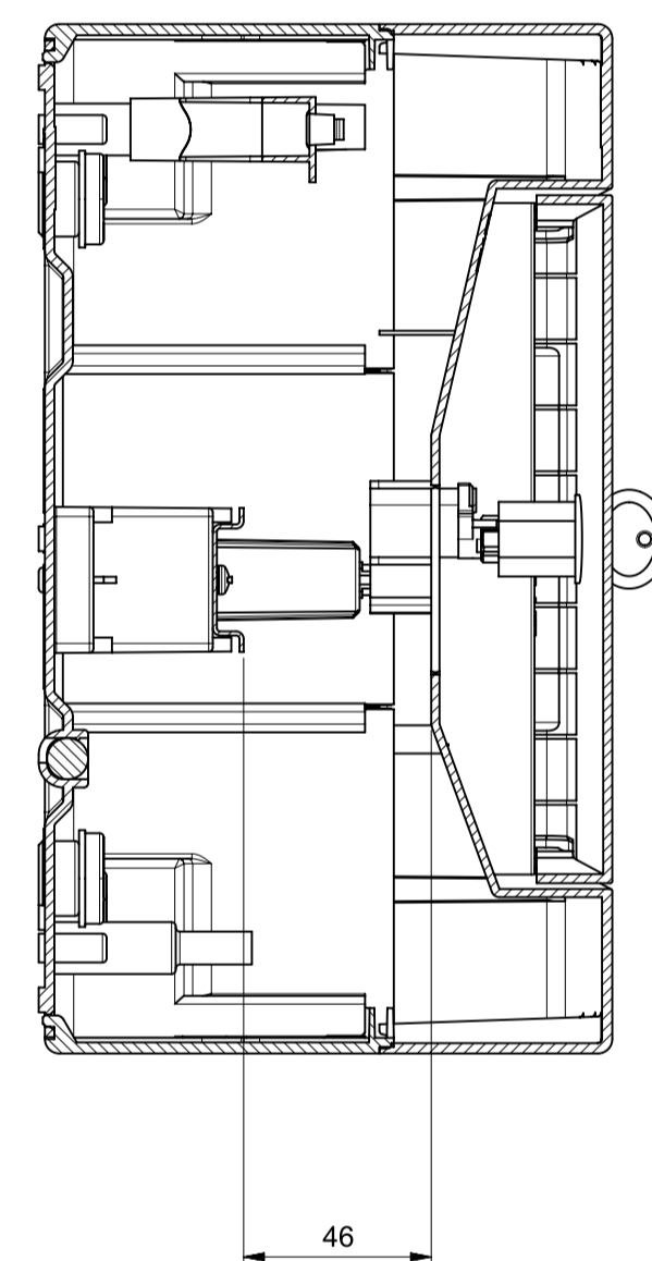
Sezione A-A
