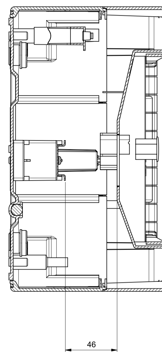
Sezione A-A
