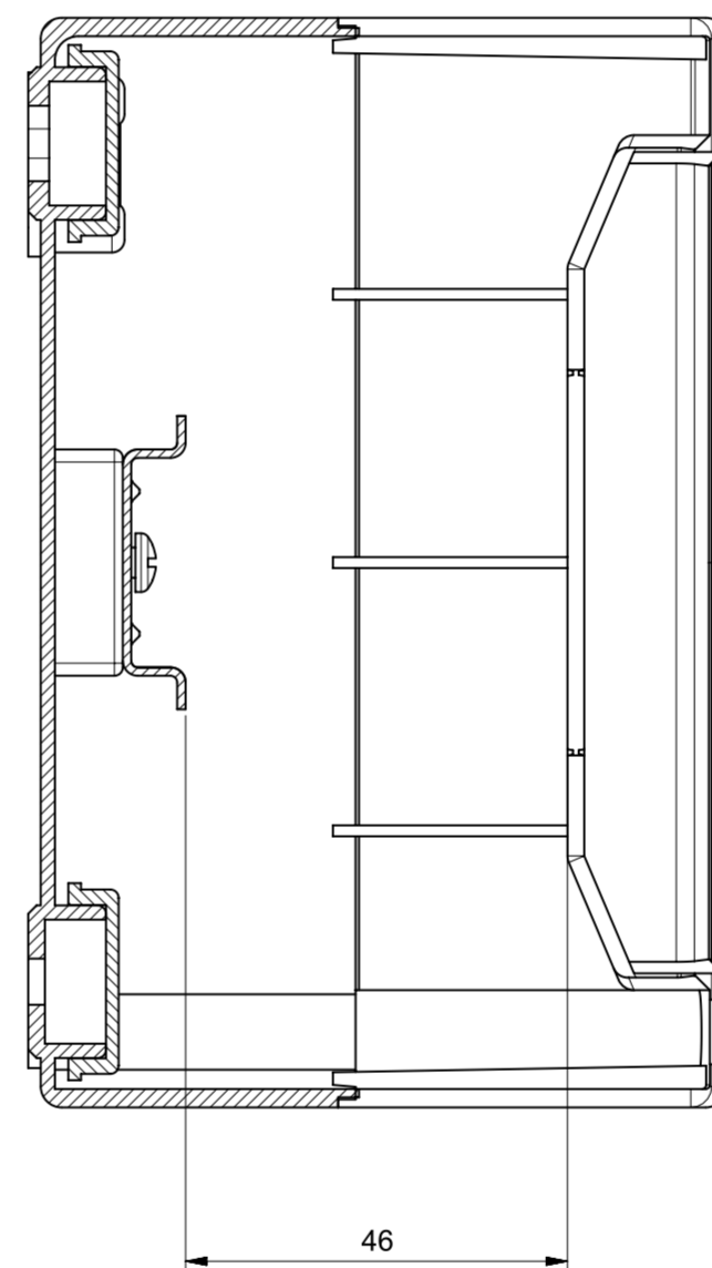
Sezione A-A
