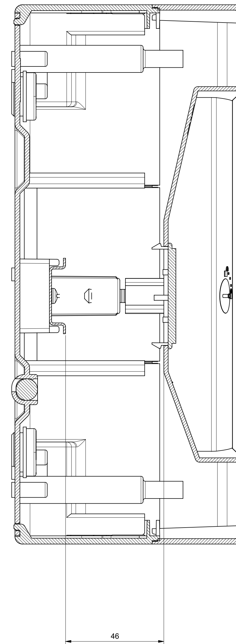
Sezione A-A
