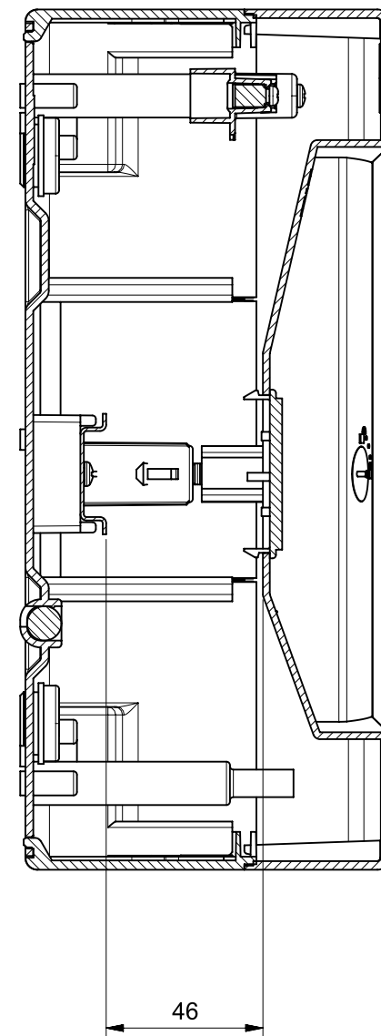
Sezione A-A
