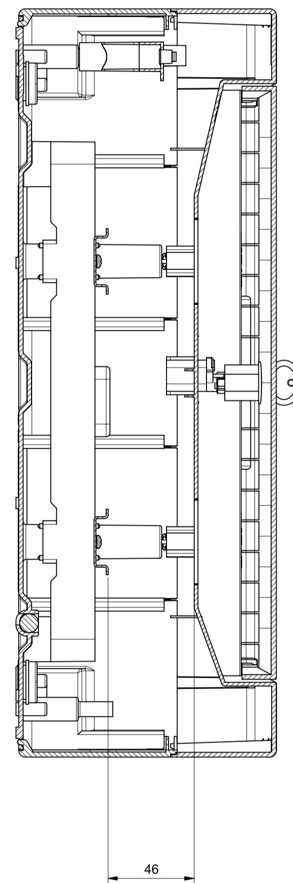
Sezione A-A
