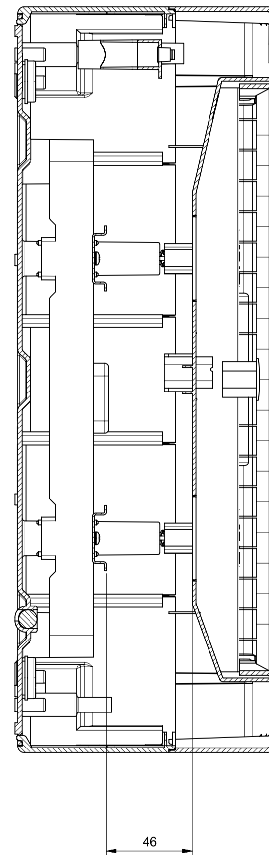
Sezione A-A
