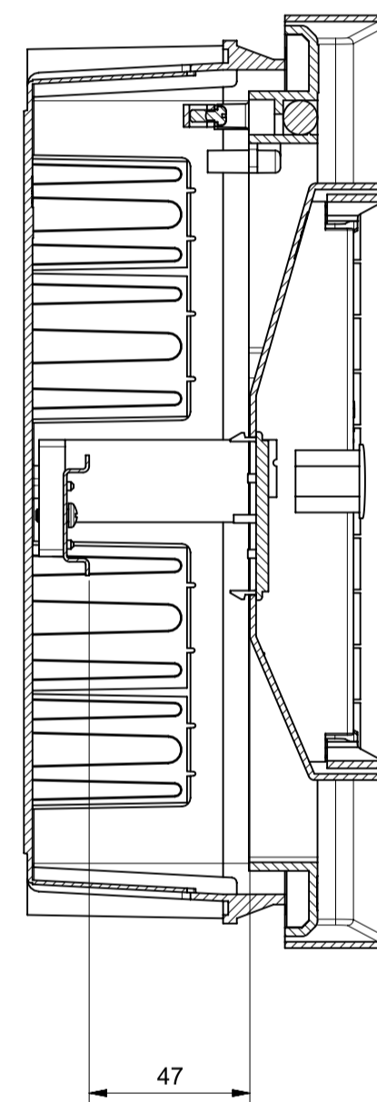
Sezione A-A
