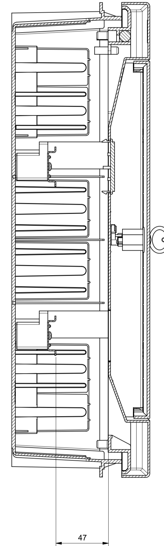
Sezione A-A
