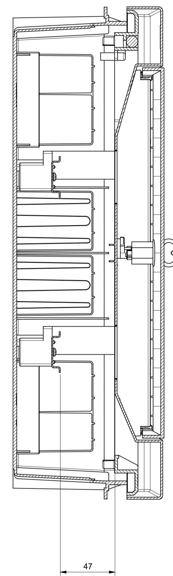
Sezione A-A
