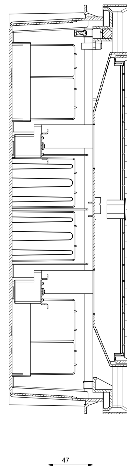
Sezione A-A
