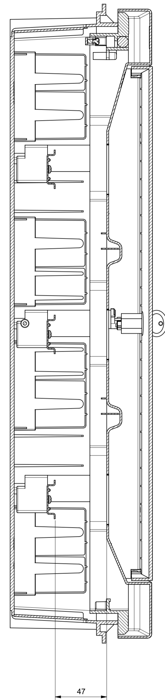
Sezione A-A
