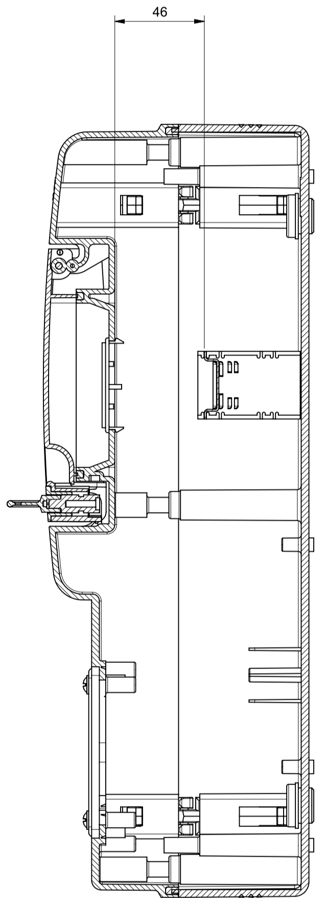
Sezione A-A
