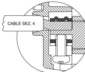
SCALA 2:1
