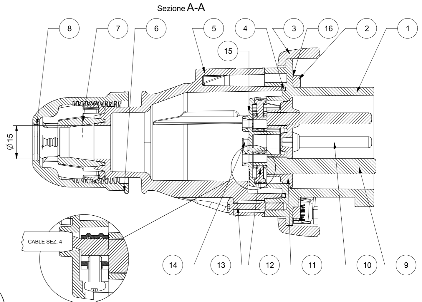
SCALA 2:1
