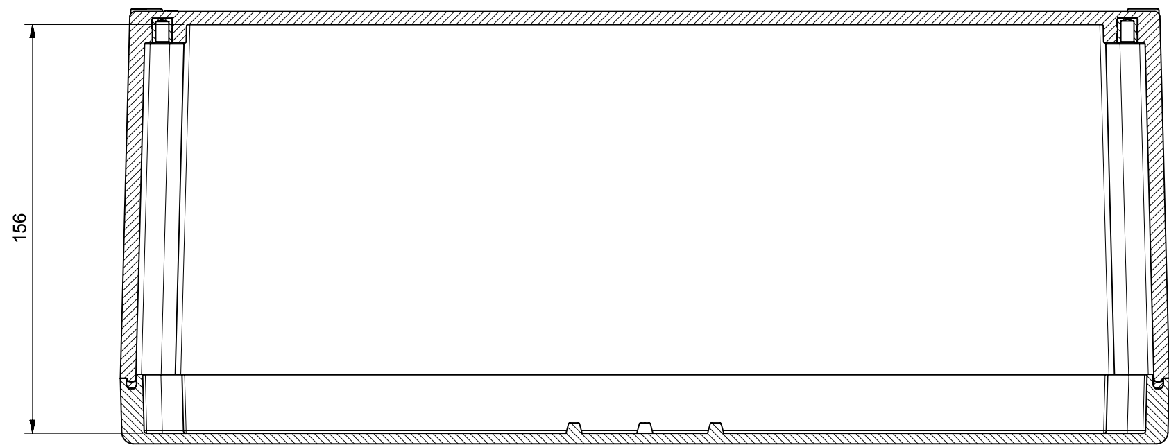
Sezione A-A
