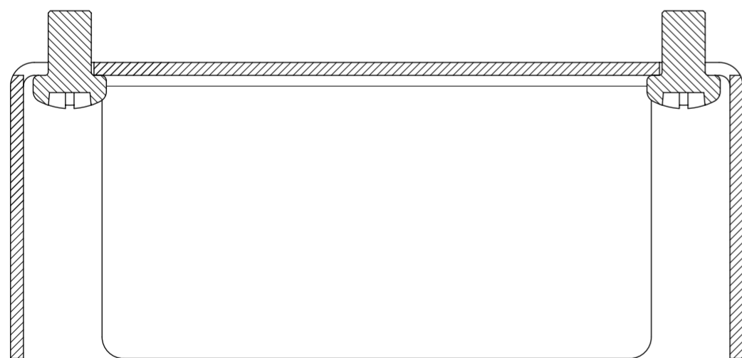
Sezione A-A
