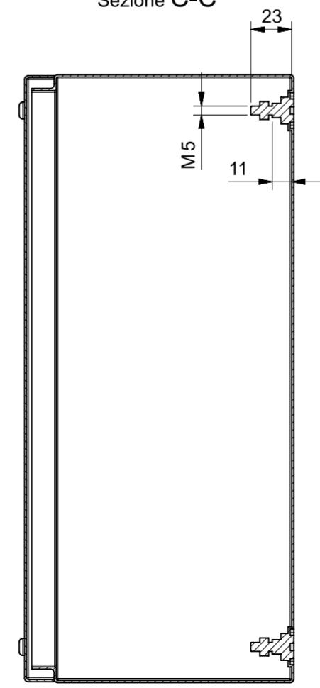
Sezione C-C
