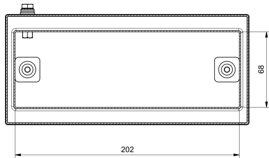
Sezione B-B
