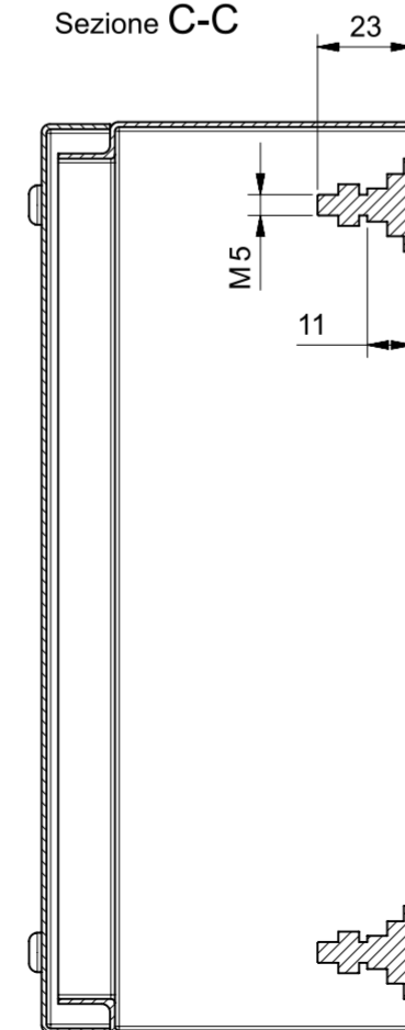
Sezione C-C
