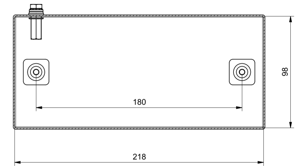
Sezione A-A
