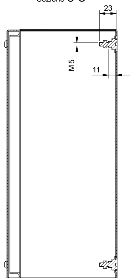
Sezione C-C
