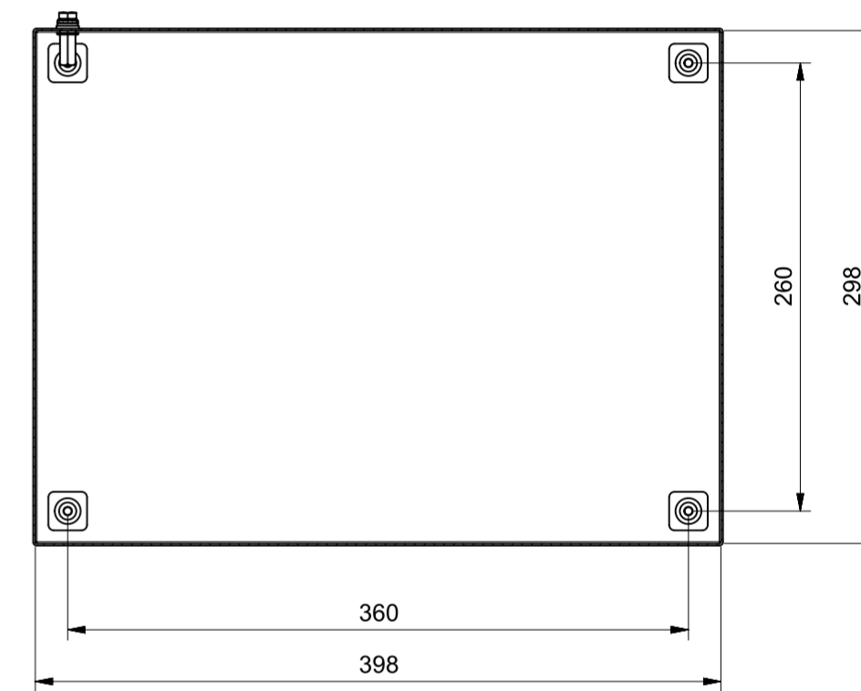
Sezione B-B
