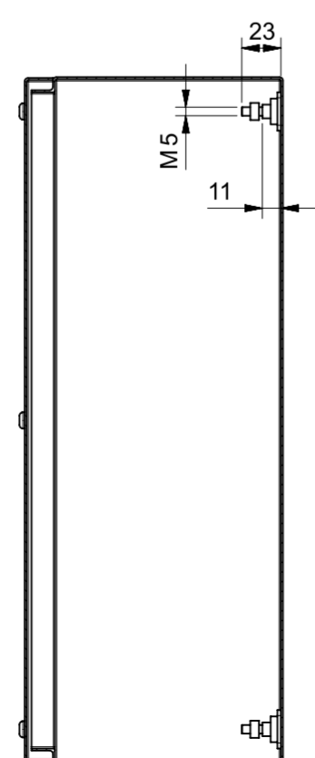
Sezione C-C
