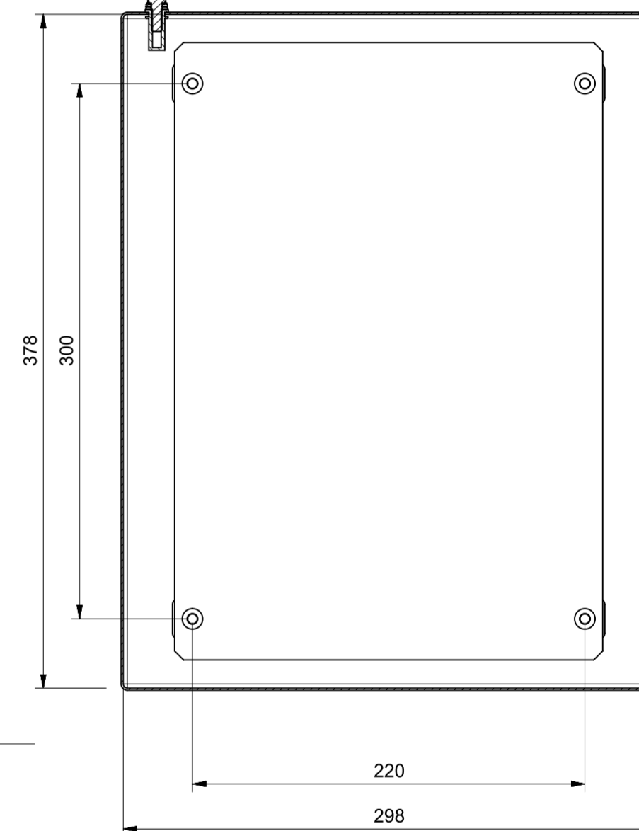
Sezione C-C
