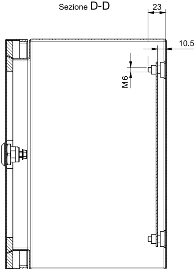
Sezione D-D
