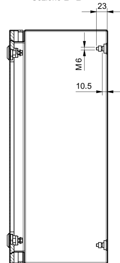
Sezione D-D
