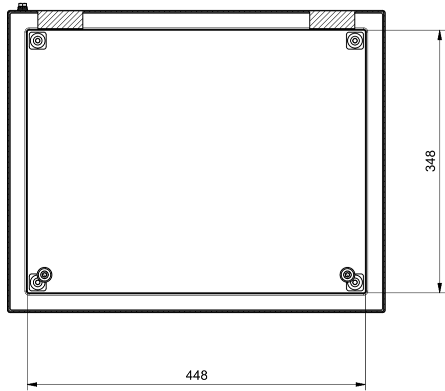
Sezione E-E
