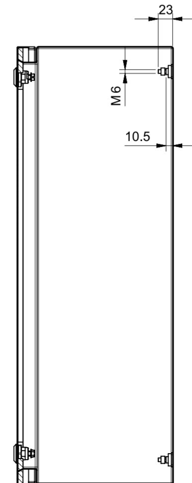
Sezione E-E
