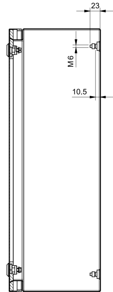
Sezione E-E
