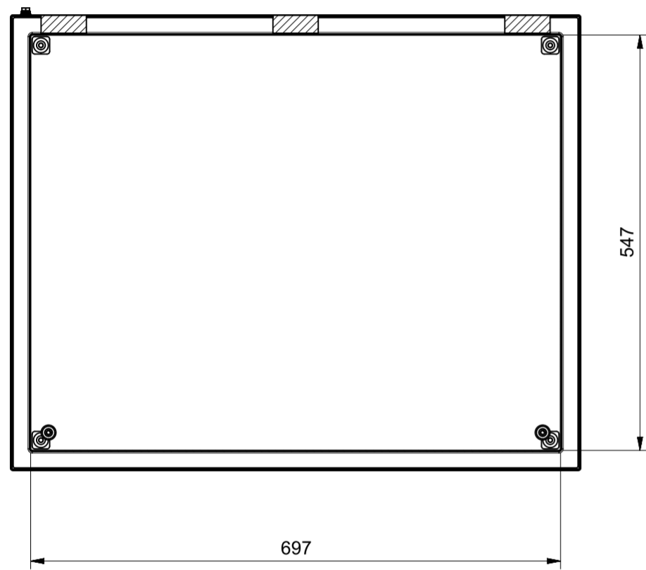
Sezione D-D
