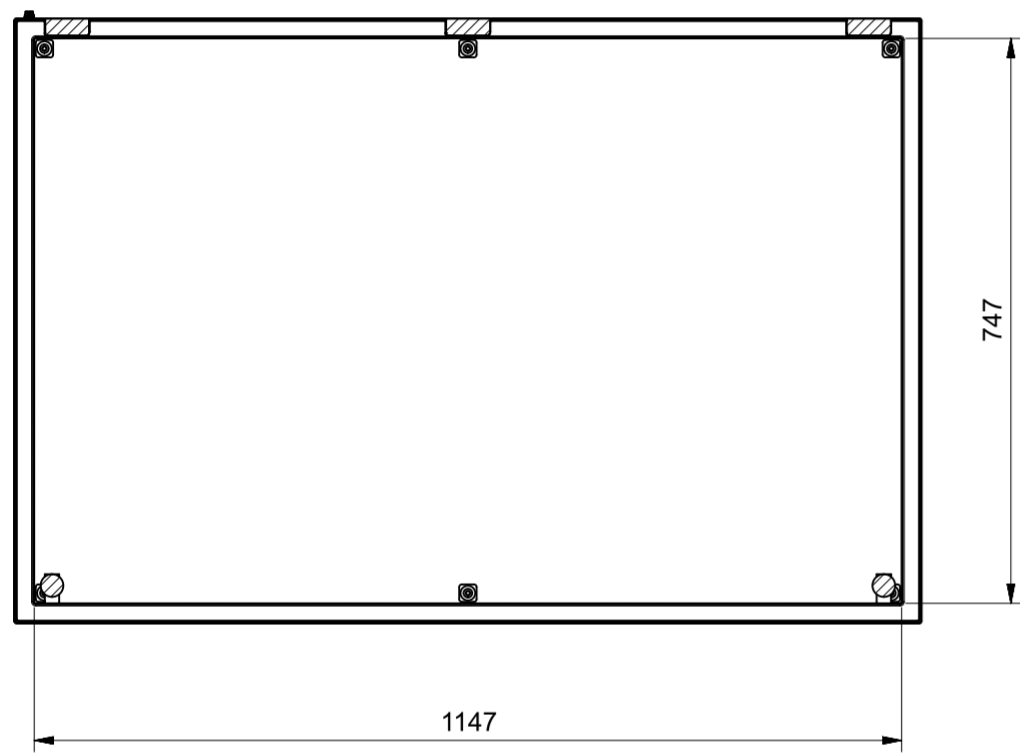
Sezione D-D
