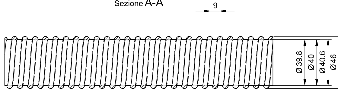
Sezione A-A
