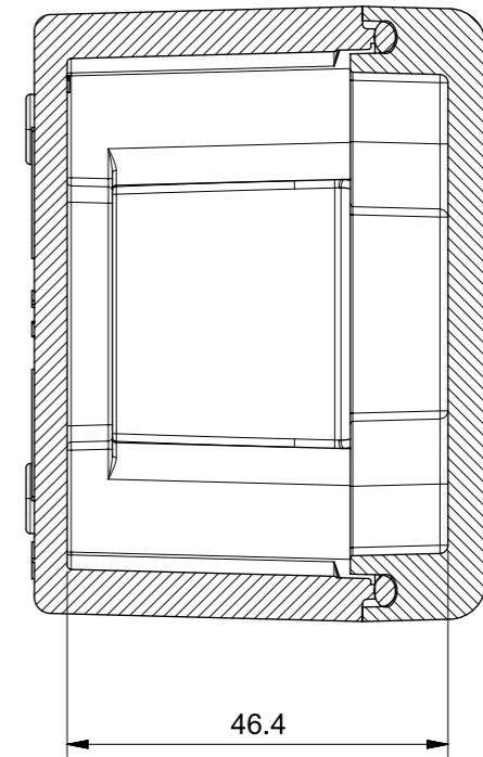
Sezione A-A
