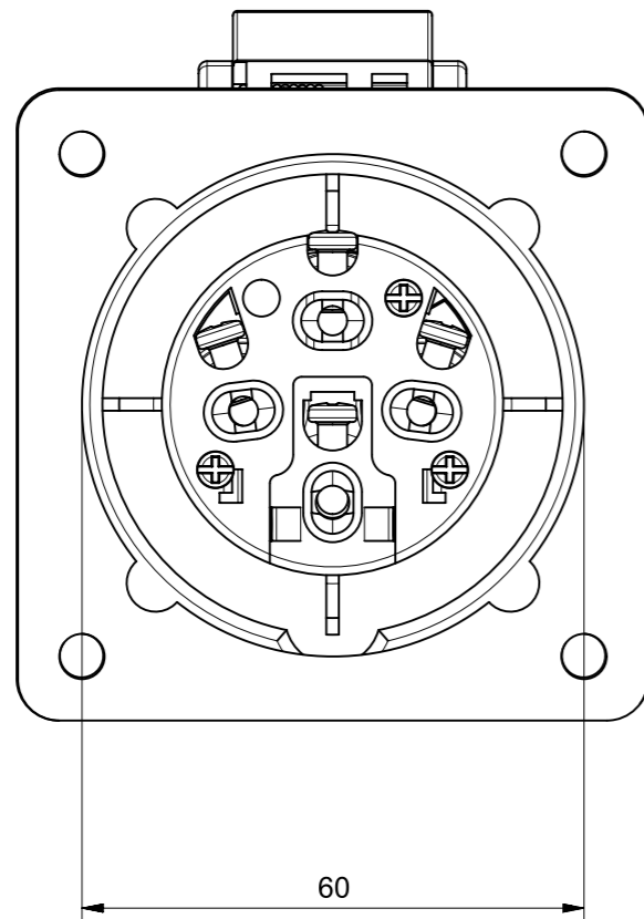
DIAMETRO DI FORATURA PANNELLO PANEL DRILLING HOLE
