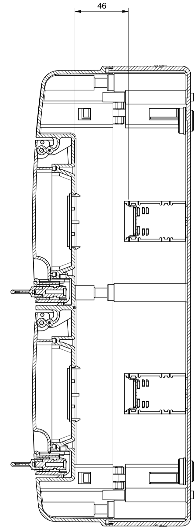
Sezione A-A
