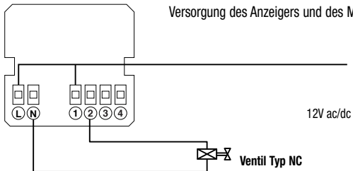
Versorgung des Anzeigers und des Magnetventils mit 12V
