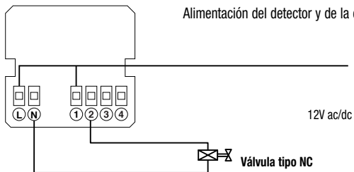
Alimentación del detector y de la electroválvula de 12V
