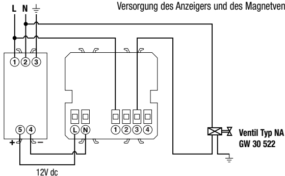
Versorgung des Anzeigers und des Magnetventils mit 230V
