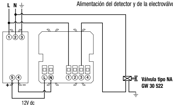
Alimentación del detector y de la electroválvula de 230V
