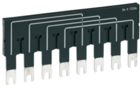
Busbar legatura 4P, HIC 63-125A
