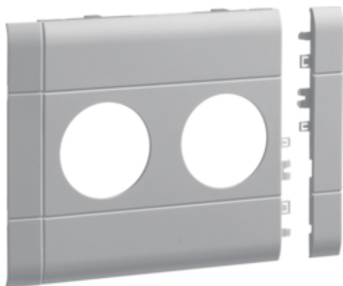
Masca dubla fara halogen, 120mm, gri, BR
