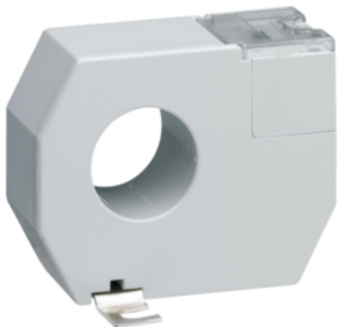
Tor circular diametru 210mm
