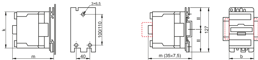
Fixare pe placă de montaj
