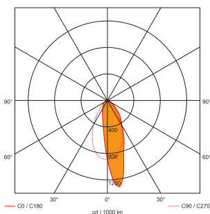
Curba fotometrică RHISA
