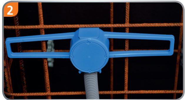
2 Für mehr als 20 mm Betondeckung die Dose einfach umdrehen.
