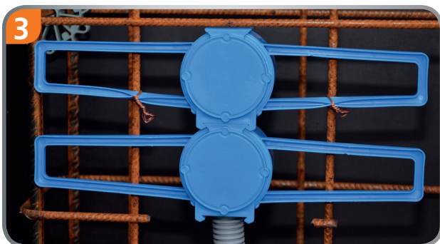
3 Bei Kombinationen feste Verbindung durch bewährte Schiebetechnik.
