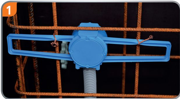
1 Rohr einführen und einfach auf die Stahlarmierung binden.
