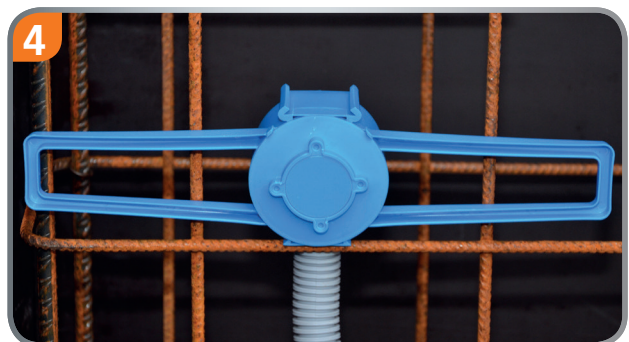
4 Auch als Leuchtauslassdose Ø 35 mm lieferbar.
