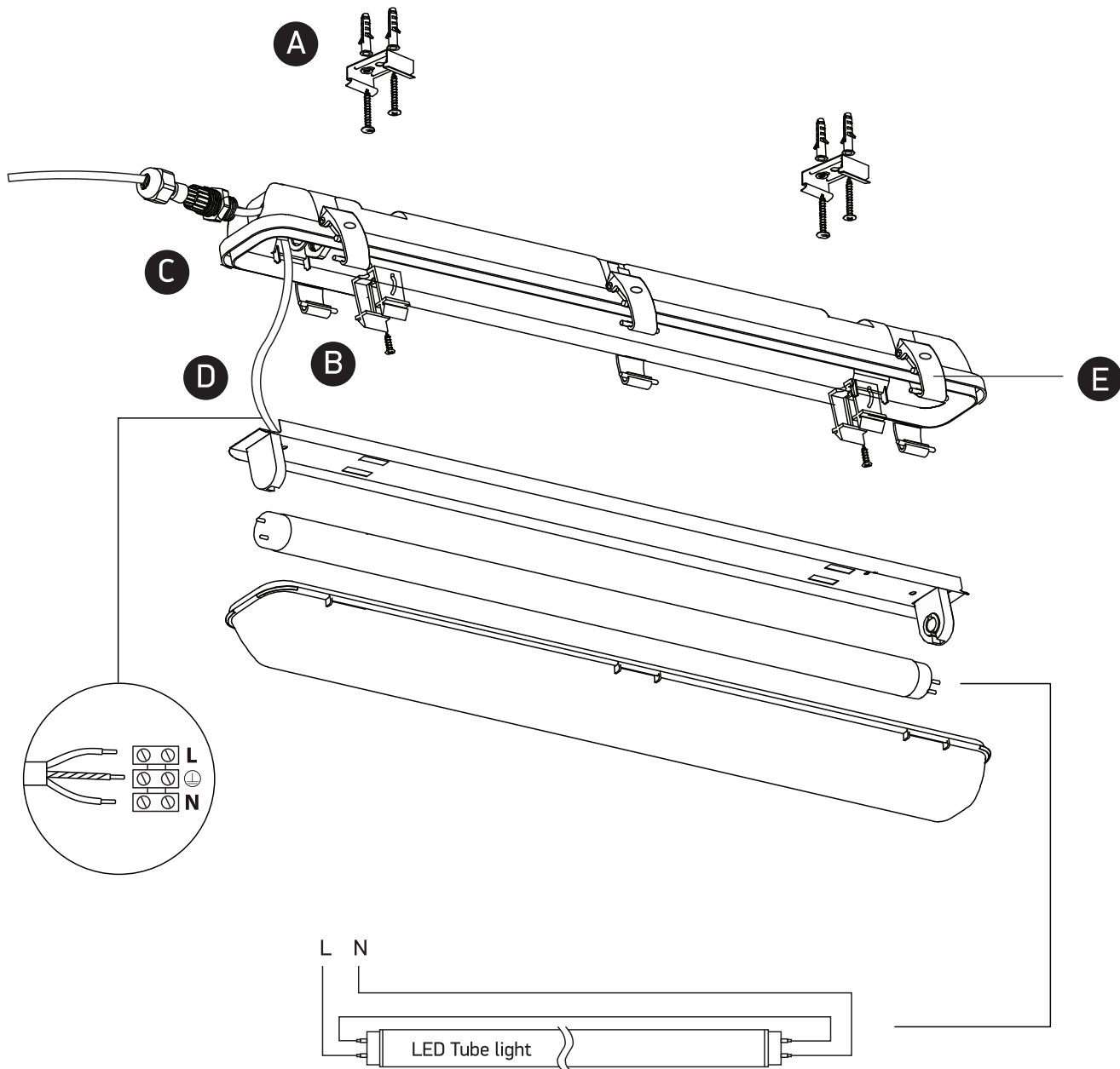
Wiring diagram.
