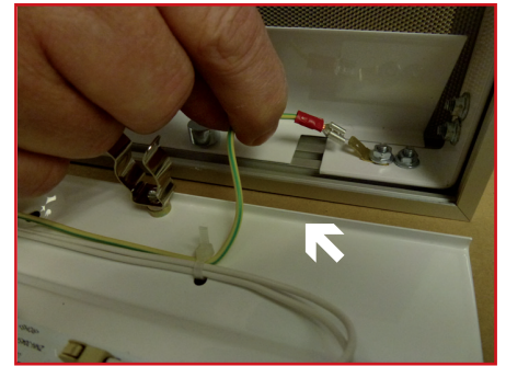
3. Erdkontakt abschalten / disconnect earthing contact
