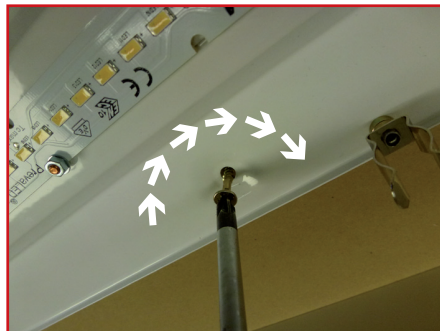
5. Mit 4 Schrauben befestigen / fix it with 4 screws
