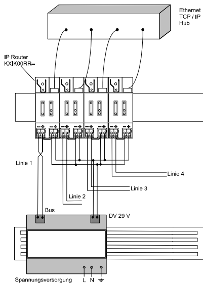
Anschlussbild 2 mit Hilfsspannungsversorgung aus unverdrosselter Busspannungsversorgung Example of Operation 2 with auxiliary power supply from unchoked bus power supply
