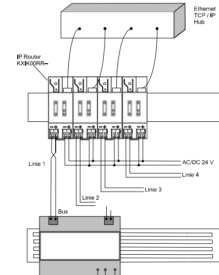
Anschlussbild 1 mit externer Hilfsspannungsversorgung Example of Operation 1 with external auxiliary power supply
