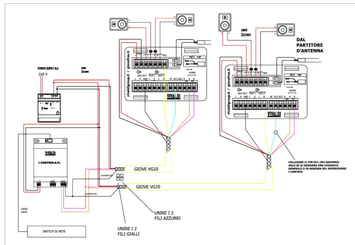
COLLEGAMENTO GIOVE FREE CON SUPERVISORE (FREECONTROL, ICONTROL4.1L, ICONTROL4.0+, EVO.VISION)
