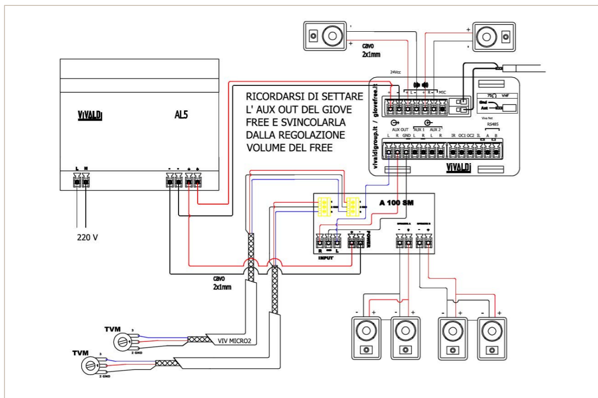
COLLEGAMENTO GIOVE FREE CON ESPANSIONE PER SUBZONA A100SM
