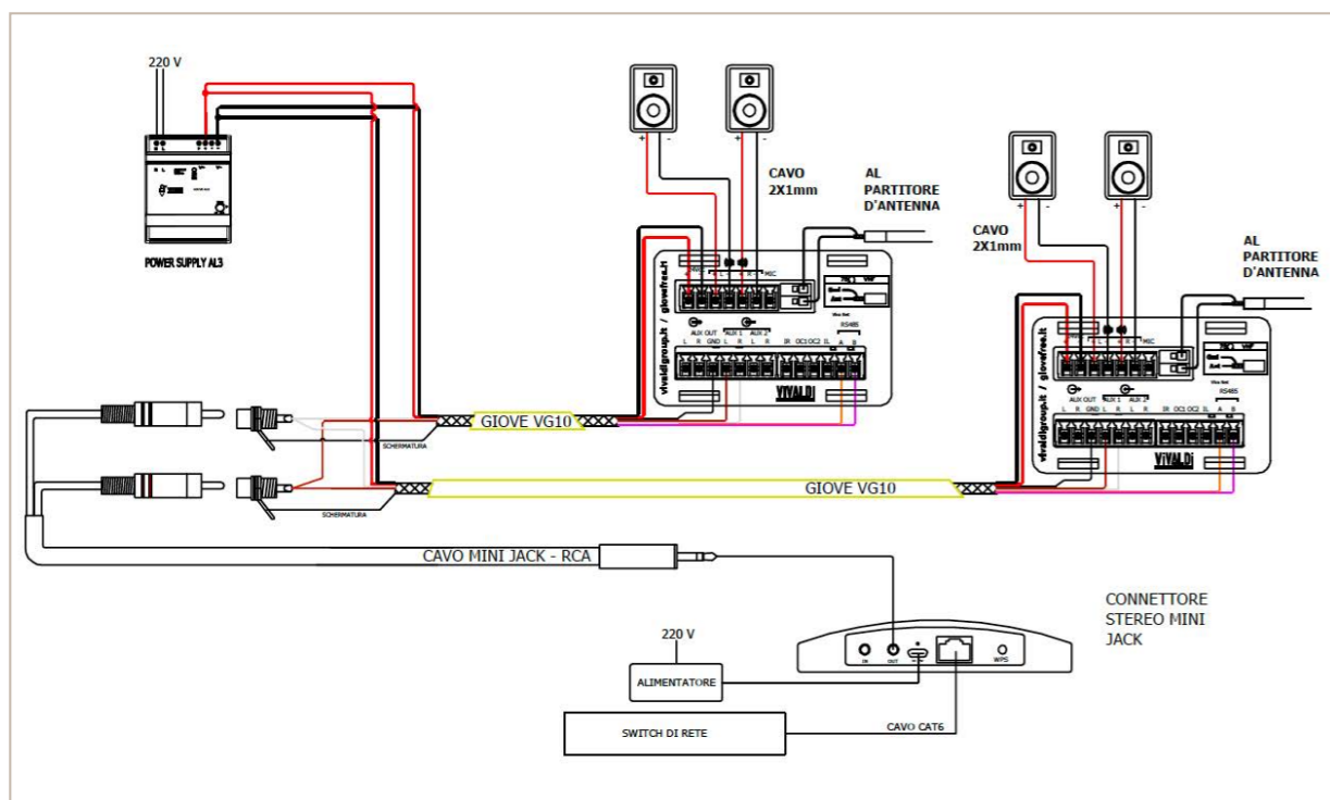
COLLEGAMENTO GIOVE FREE CON KEYSOL TRAMITE IL CAVO VIVALDI VG10
