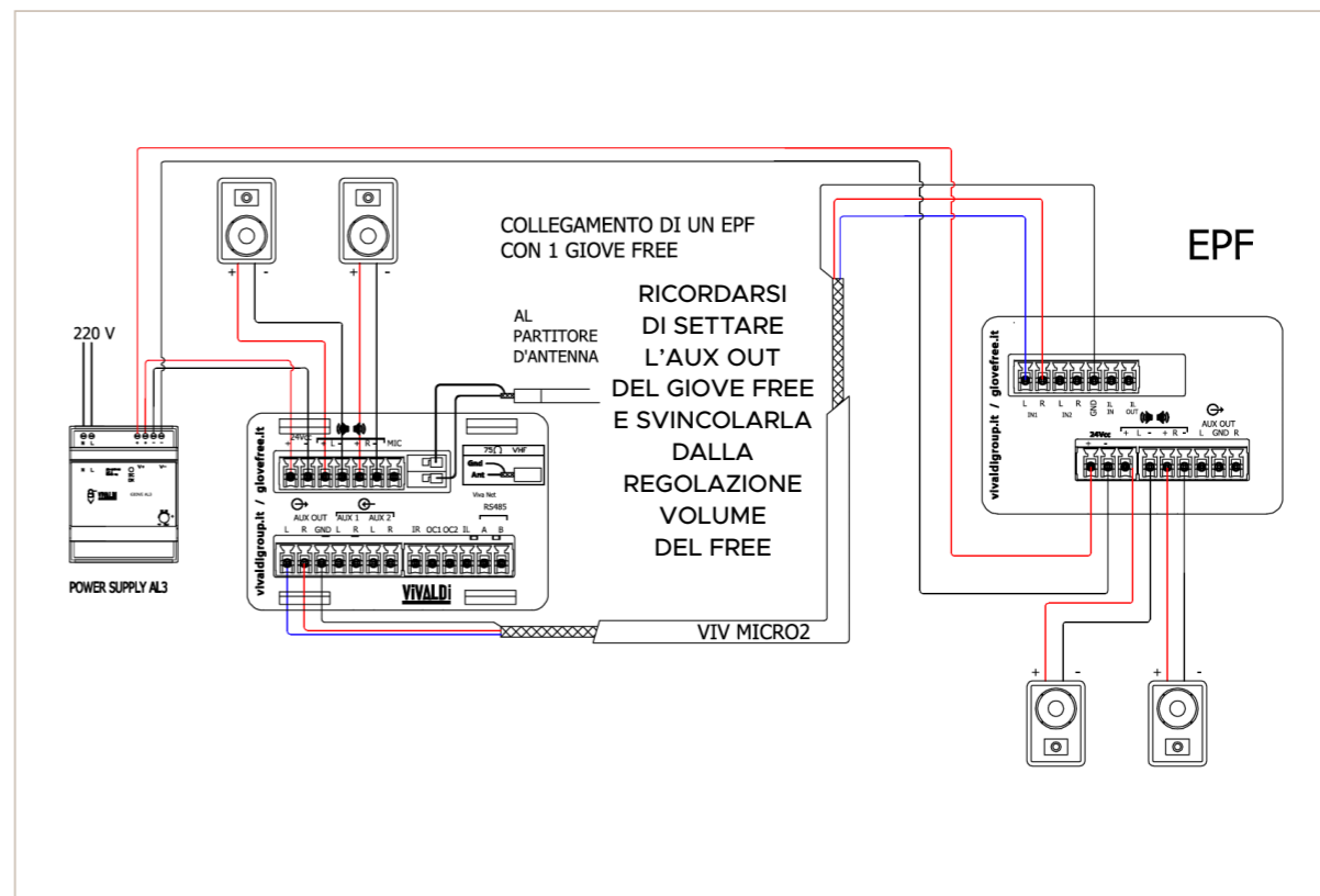
COLLEGAMENTO GIOVE FREE CON ESPANSIONE PER SUBZONA EPF
