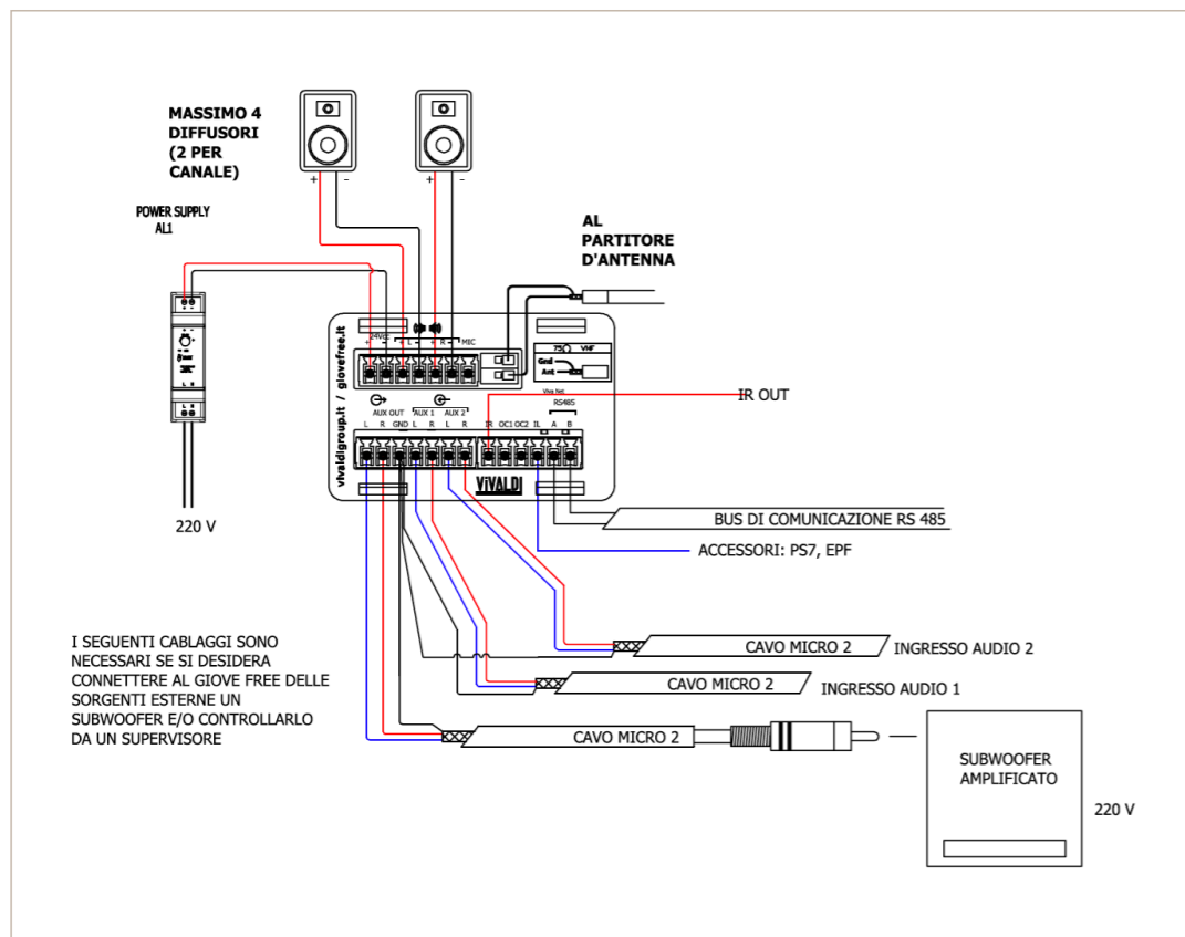
COLLEGAMENTO GIOVE FREE CON SORGENTI ESTERNE E SUBWOOFER
