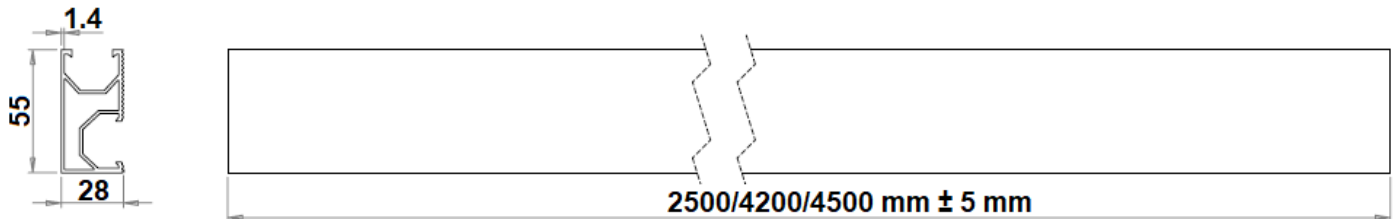
Fig. 1 - Dimensiuni bara sustinere
