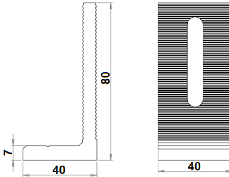
Fig. 1 - Clema L Feet - dimensiuni
