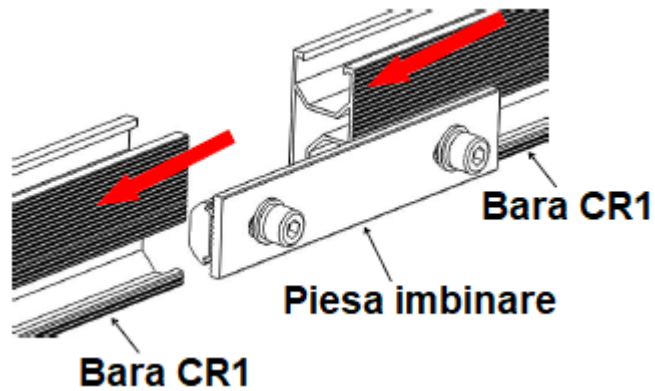
Fig. 1 - Imbinare bare CR1
