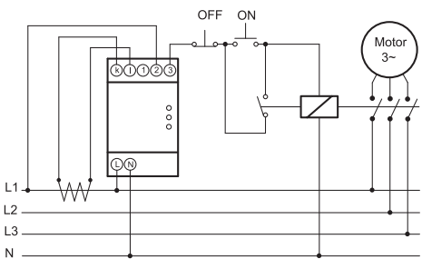
Diagrame de funcționare - TFKV-AKA05
