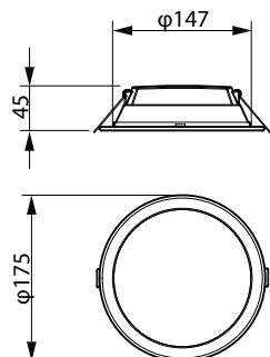
DN065B G3 LDNR LED10/840 10.5W D150 RD
